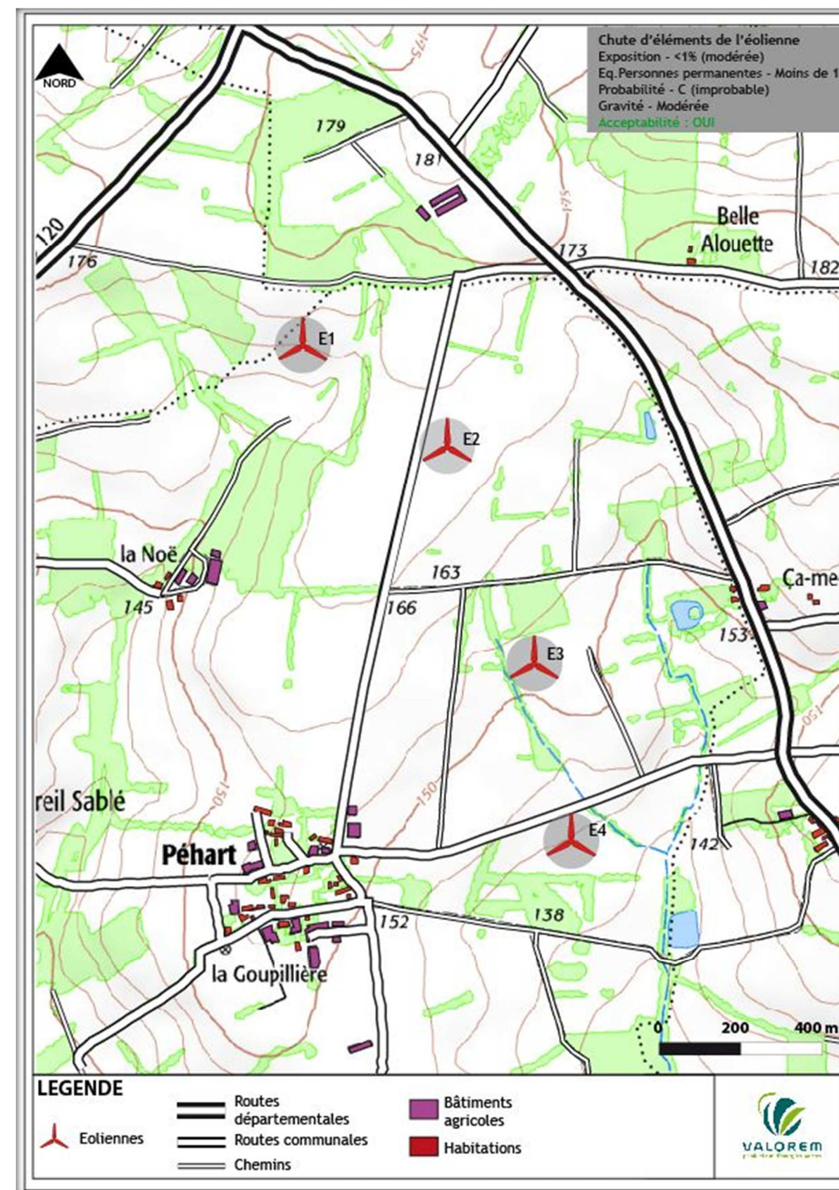
Zone d'effet du phénomène « Chute d'éléments de l'éolienne »
