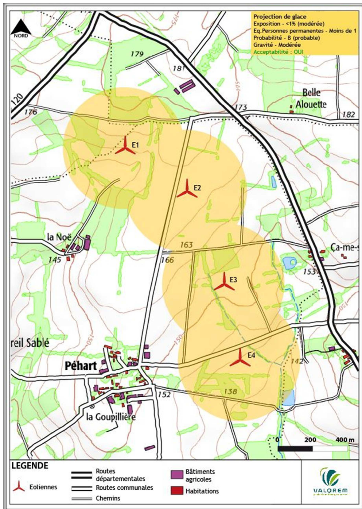
Zone d'effet du phénomène « Projection de glace »
