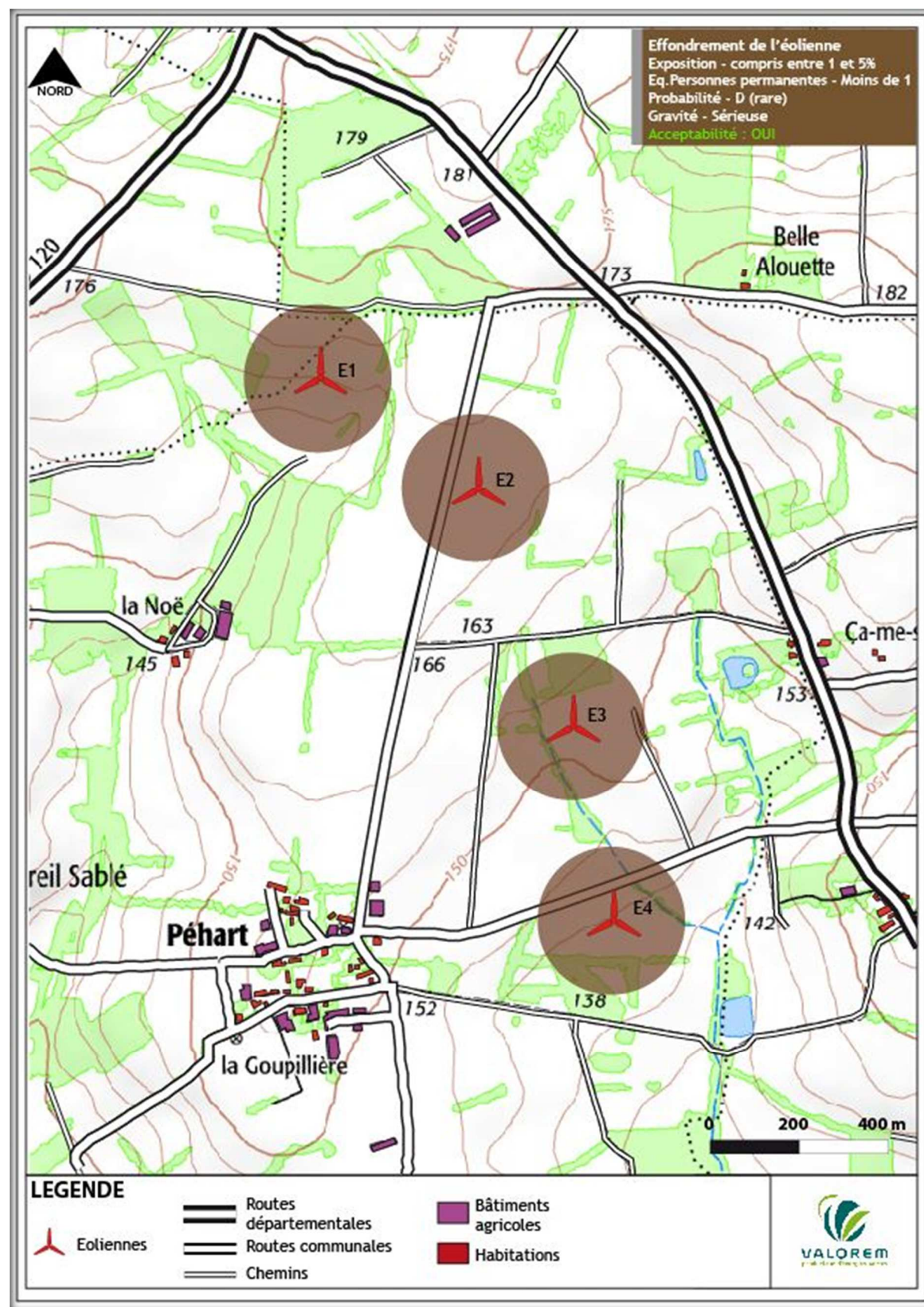
Zone d'effet du phénomène « Effondrement de l'éolienne »
