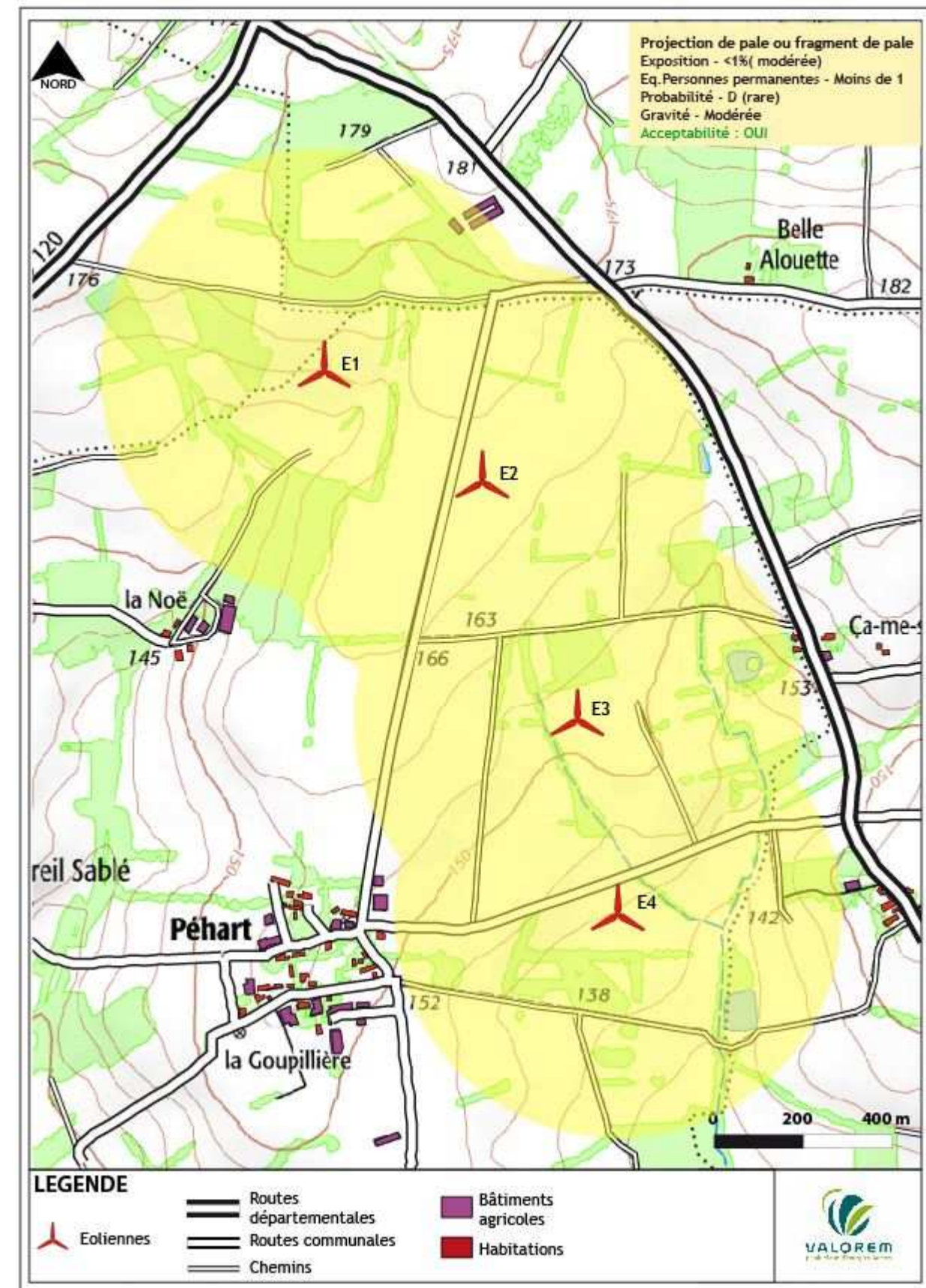
Zone d'effet du phénomène « Projection de pales ou de fragments de pales »
