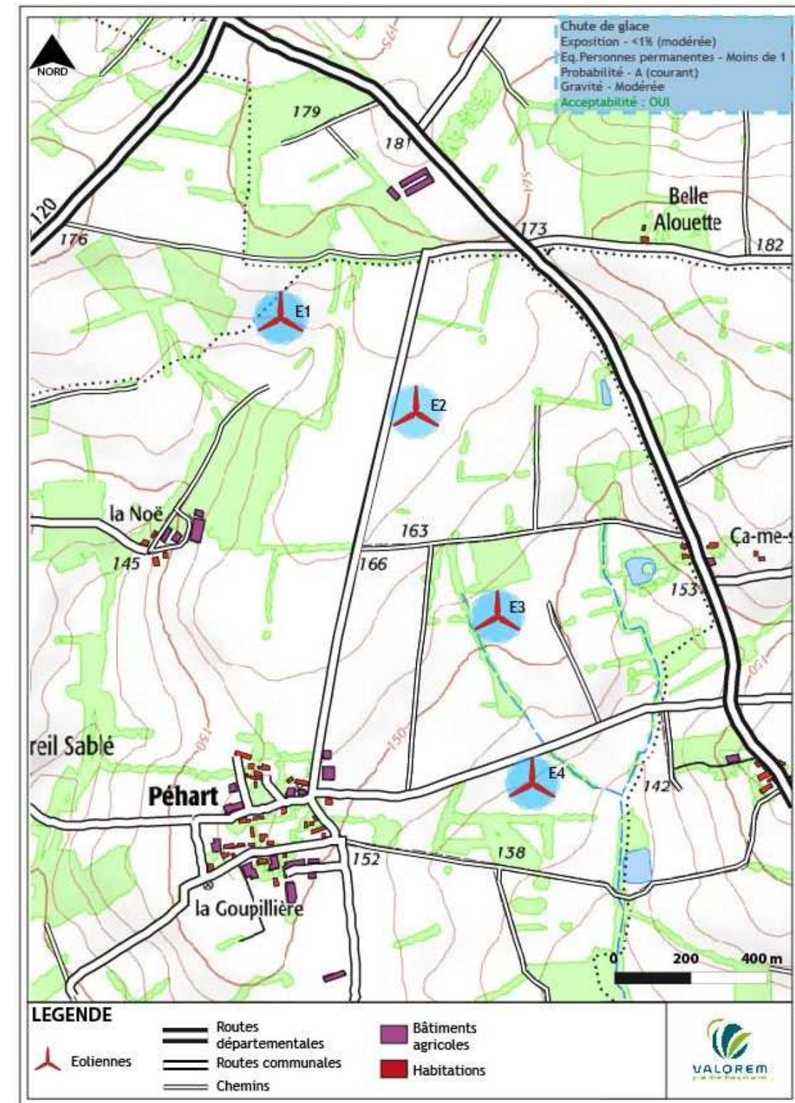
Zone d'effet du phénomène « Chute de glace » 68 mètres
